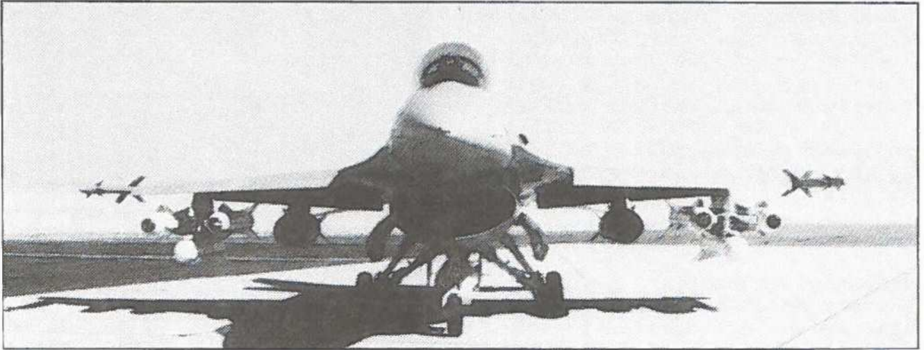
En F-16A med en blanding af TV-styrede, krigsskarpe Maverick missiler og ekscermissiler. I alt seks missiler medføres på de to LAU- 88 A/A launchers.
