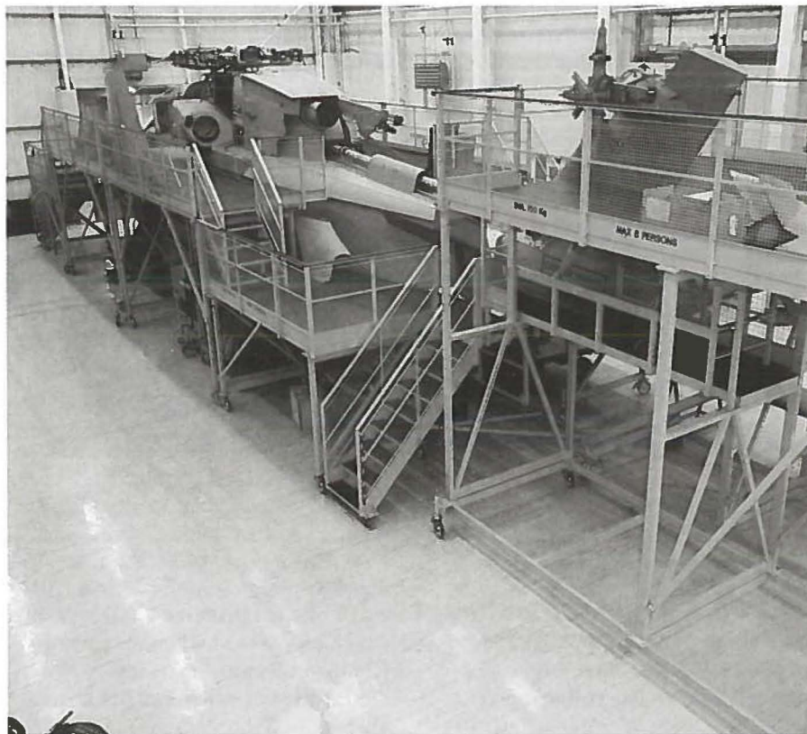
Teknikerne får deres sag for, når de skal til at fejlfinde på denne EH101, som instruktørerne kan behæfte med enhver tænkelig fejl. (Billede s-n).
