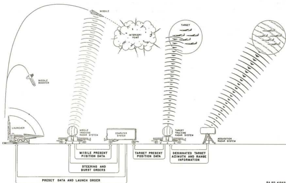
Fig. 2. Skematisk NIKE-engagement.
