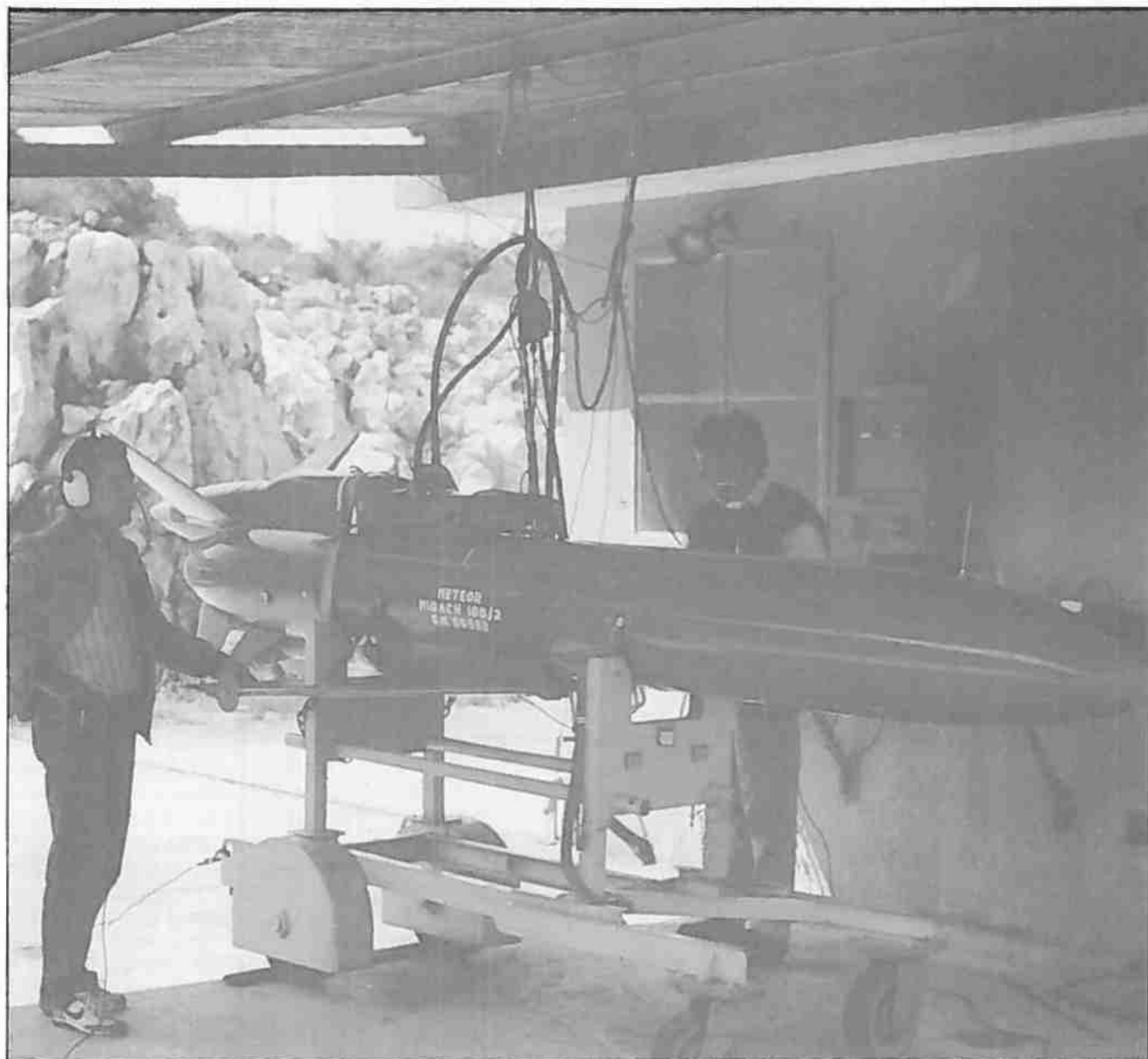
Dronen klargøres og afprøves i motorprøvestand i dagene før den skal flyve. Efter hver flyvetur lander dronen i Middelhavet med faldskærm. Den bliver samlet op med helikopter, rensat og klargjort til endnu en tur.
